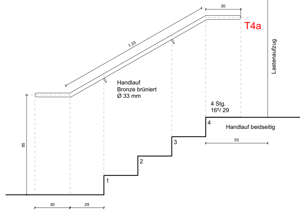
Ansicht Handlauf A - M 1:20
