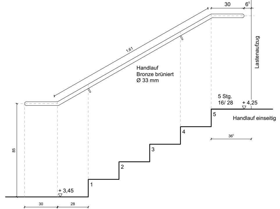
Ansicht Handlauf - M 1:20
