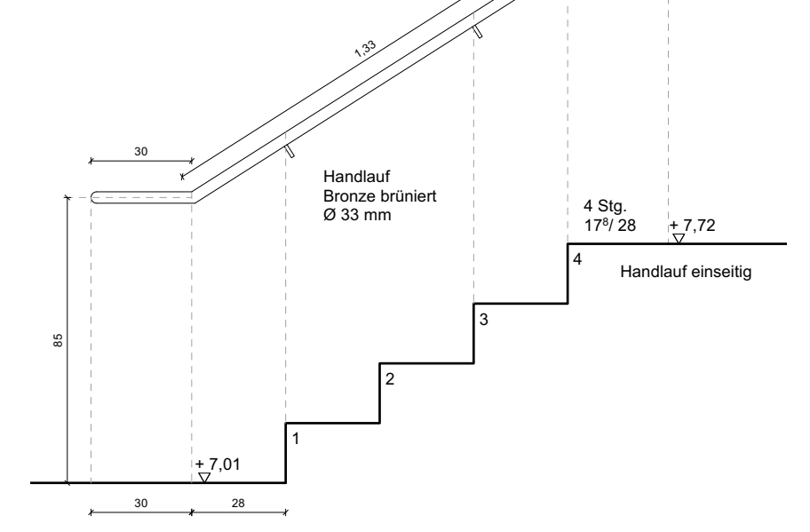
Ansicht Handlauf - M 1:20
