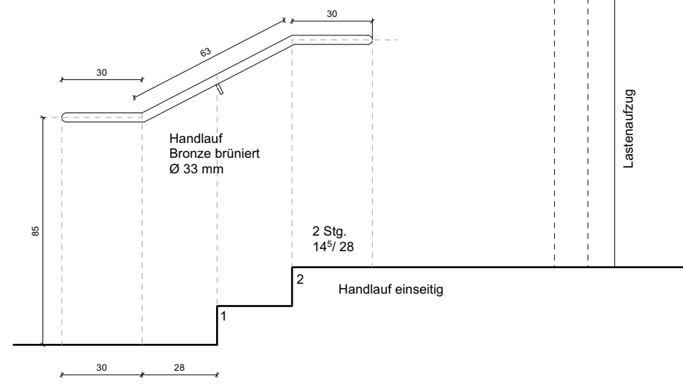
Ansicht Handlauf - M 1:20
