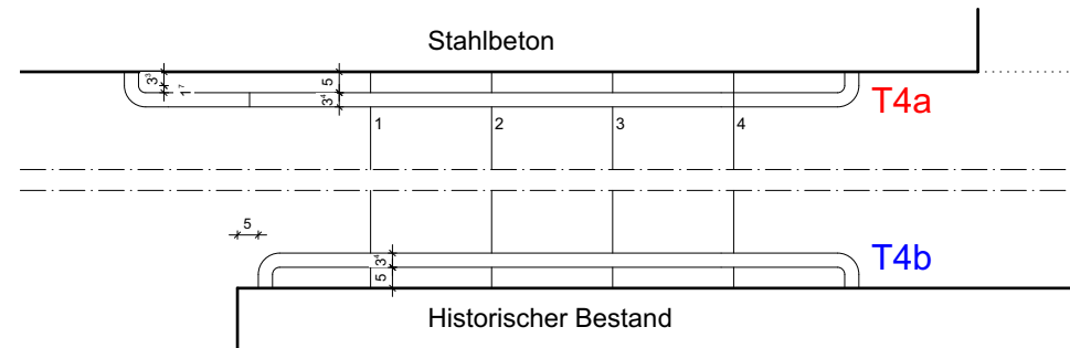
Grundriss Untergeschoss - M 1:20
